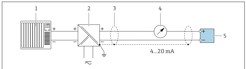
图 3 4...20 mA HART 电流输出 (无源) 的连接示例
