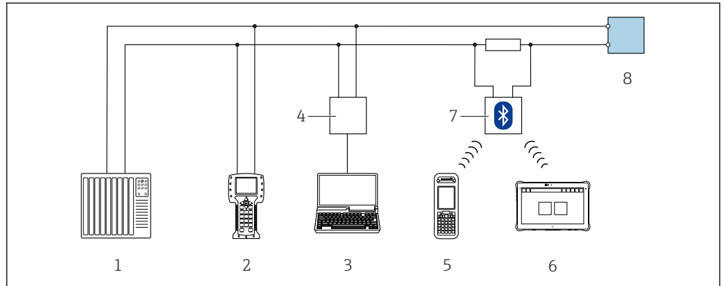
48 通过 HART 通信进行远程操作 (有源信号)
