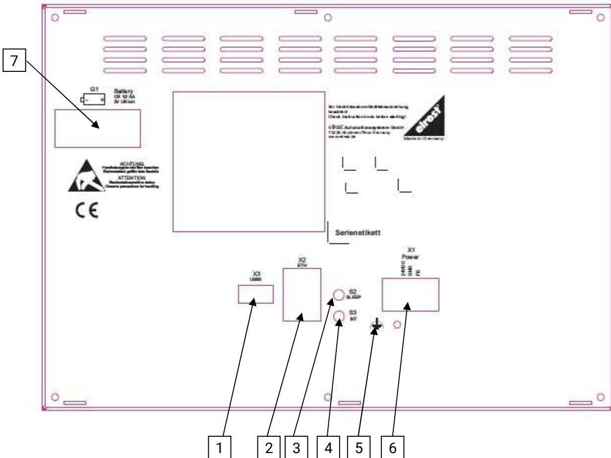
Abbildung 12: Schnittstellenrückansicht PTE510
