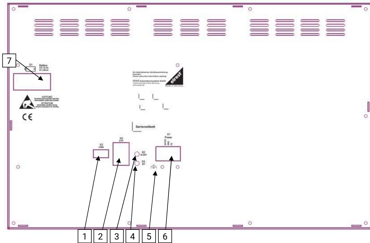
Abbildung 13: Schnittstellenrückansicht PTE715
