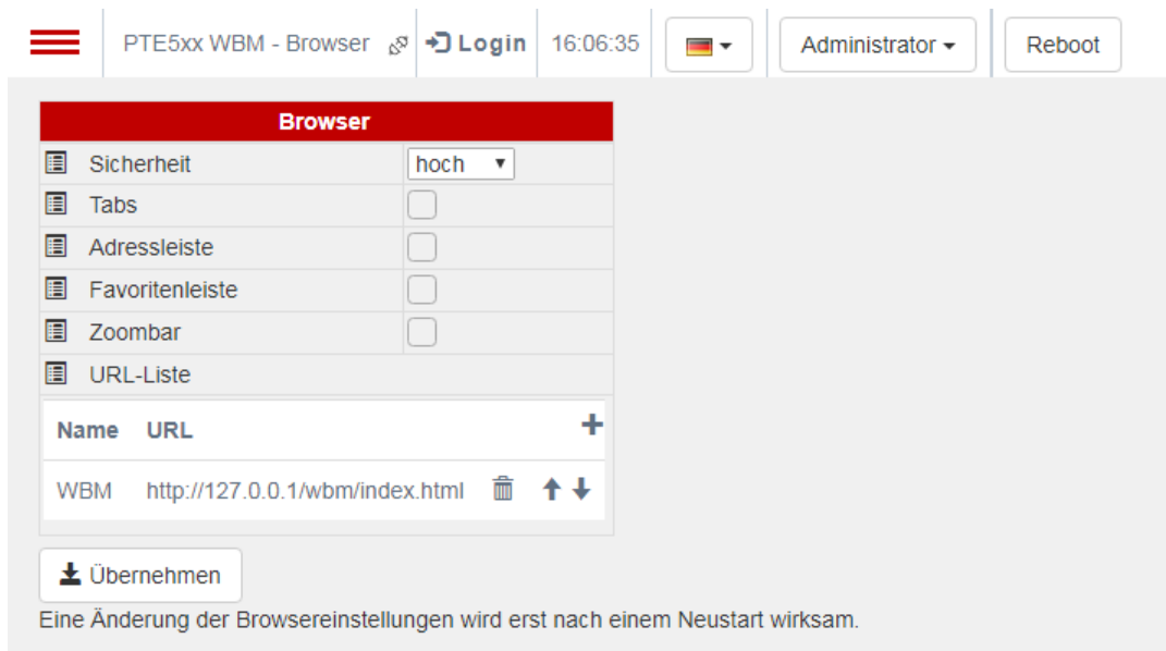
Abbildung 26: WBM – Browser
