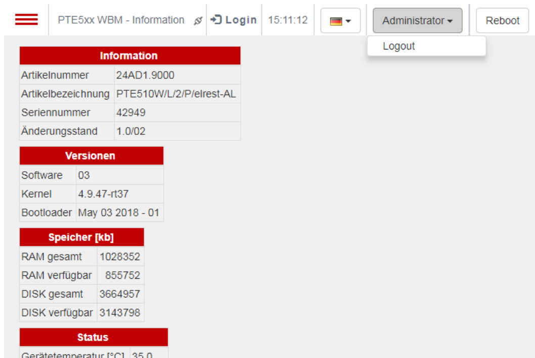
Abbildung 19: Benutzergruppen
