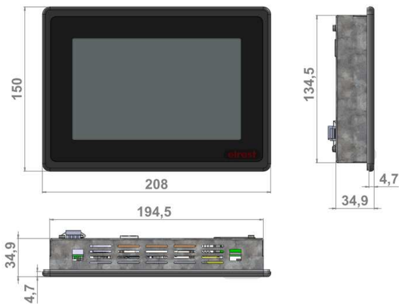
Abbildung 5: Maßzeichnung PTE507
