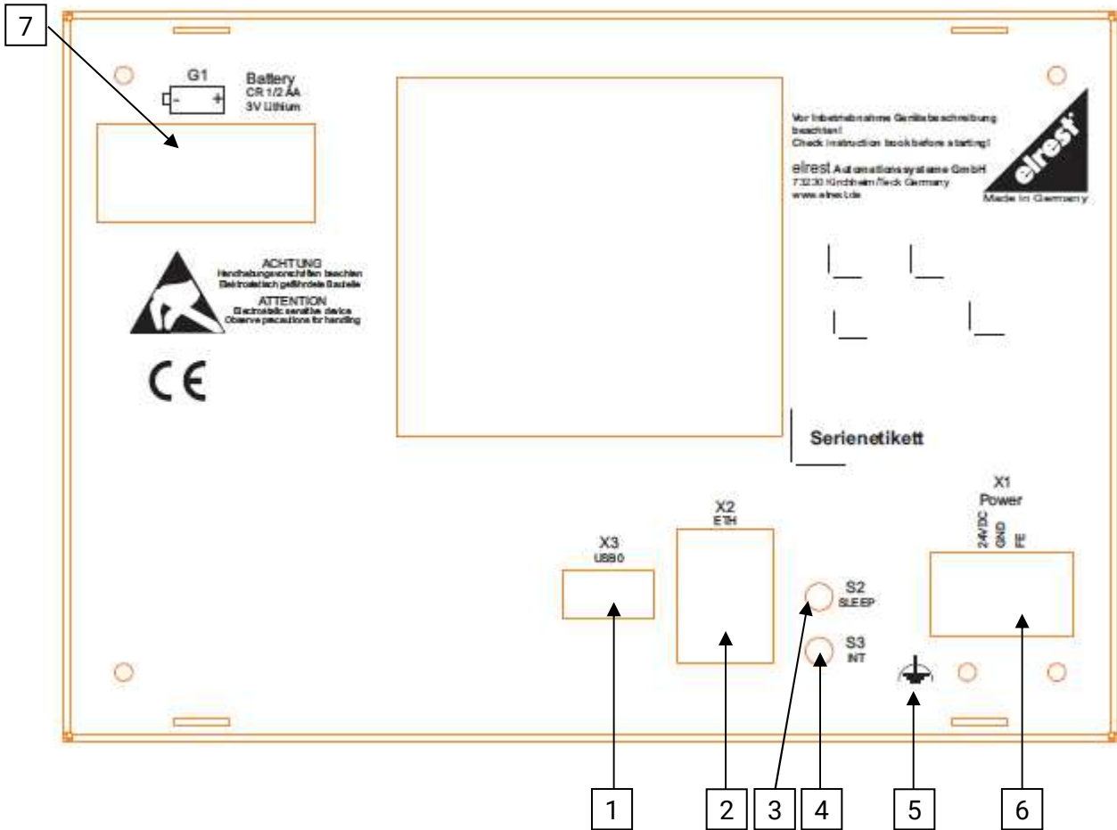
Abbildung 11: Schnittstellenrückansicht PTE507
