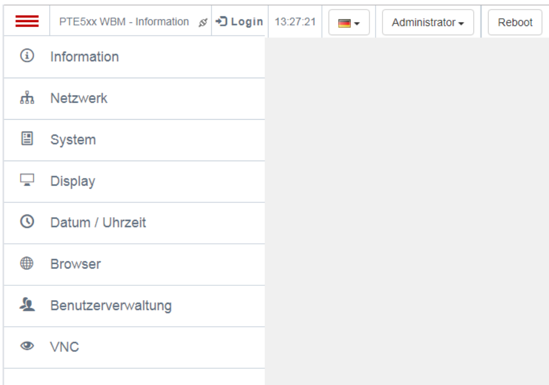
Abbildung 20: WBM Auswahlmenü
