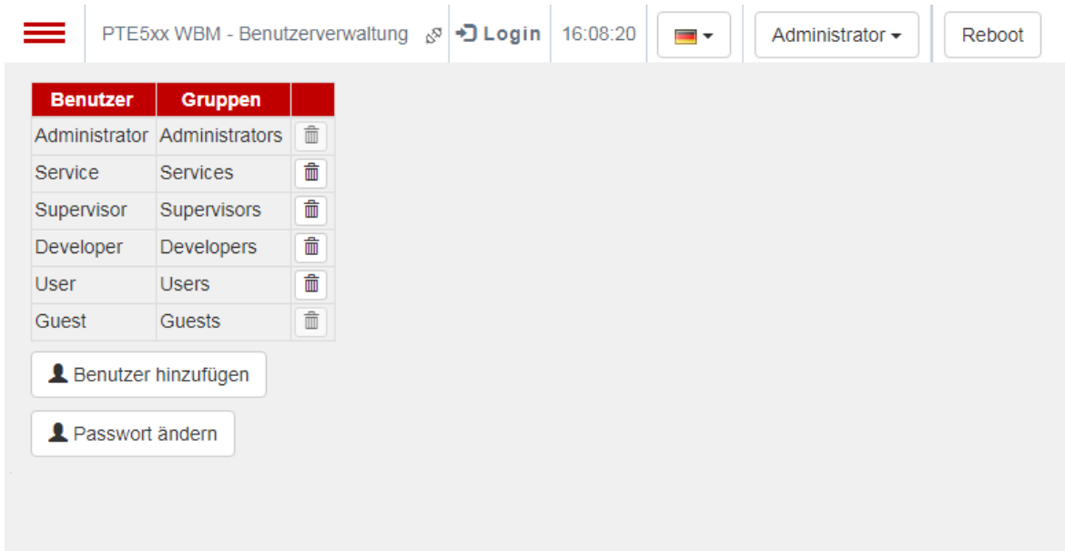
Abbildung 27: WBM – Benutzerverwaltung
