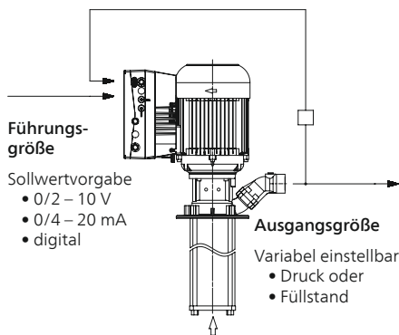
Abb. 2: Schema einer Regelung
