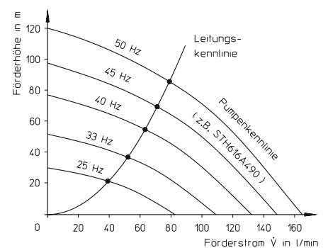
Abb. 1: Kennlinienfeld
