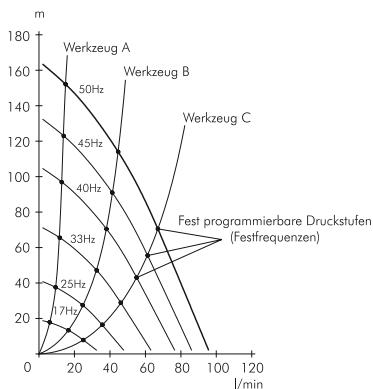
Abb. 6: Festfrequenzen
