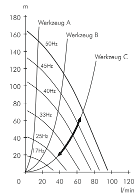
Abb. 5: Analogsignal (stufenlos)
