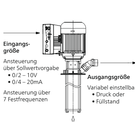
Abb. 4: Schema einer Steuerung
