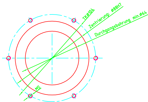
Bohrbild fuer Werkzeugaufnahme
