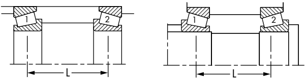
面对面安装
