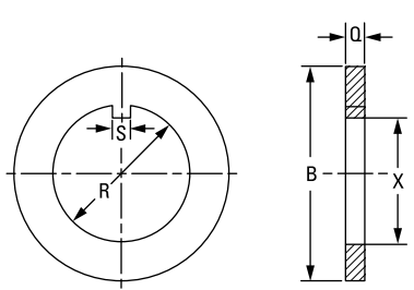
图 51. 凸缘垫圈
