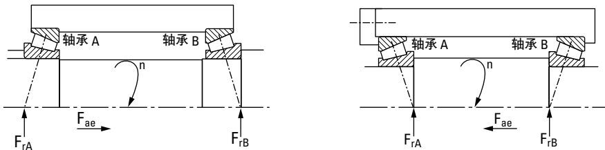
设计（外部推力 Fa 作用在轴承 A 上）
