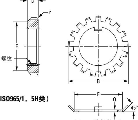
图 50. 锁紧垫圈
