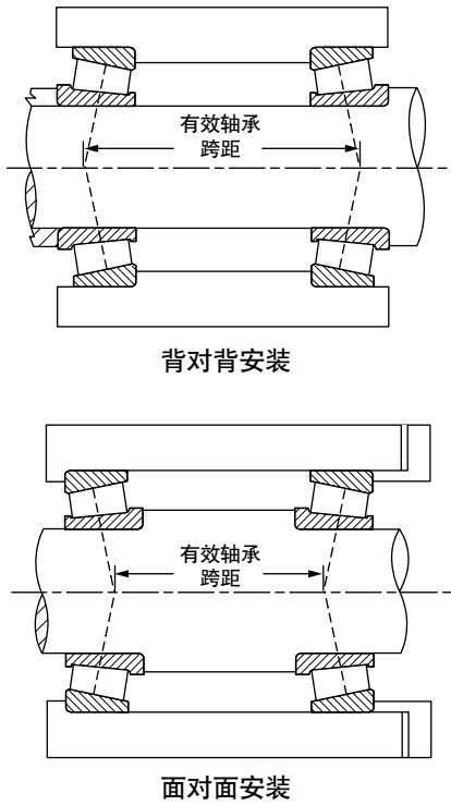
图 9. 比较面对面安装和背对背安装的稳定性
