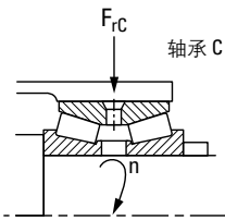
浮动轴承
