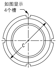
图 49. 防松螺母（螺纹符合ISO965/1，5H类）
