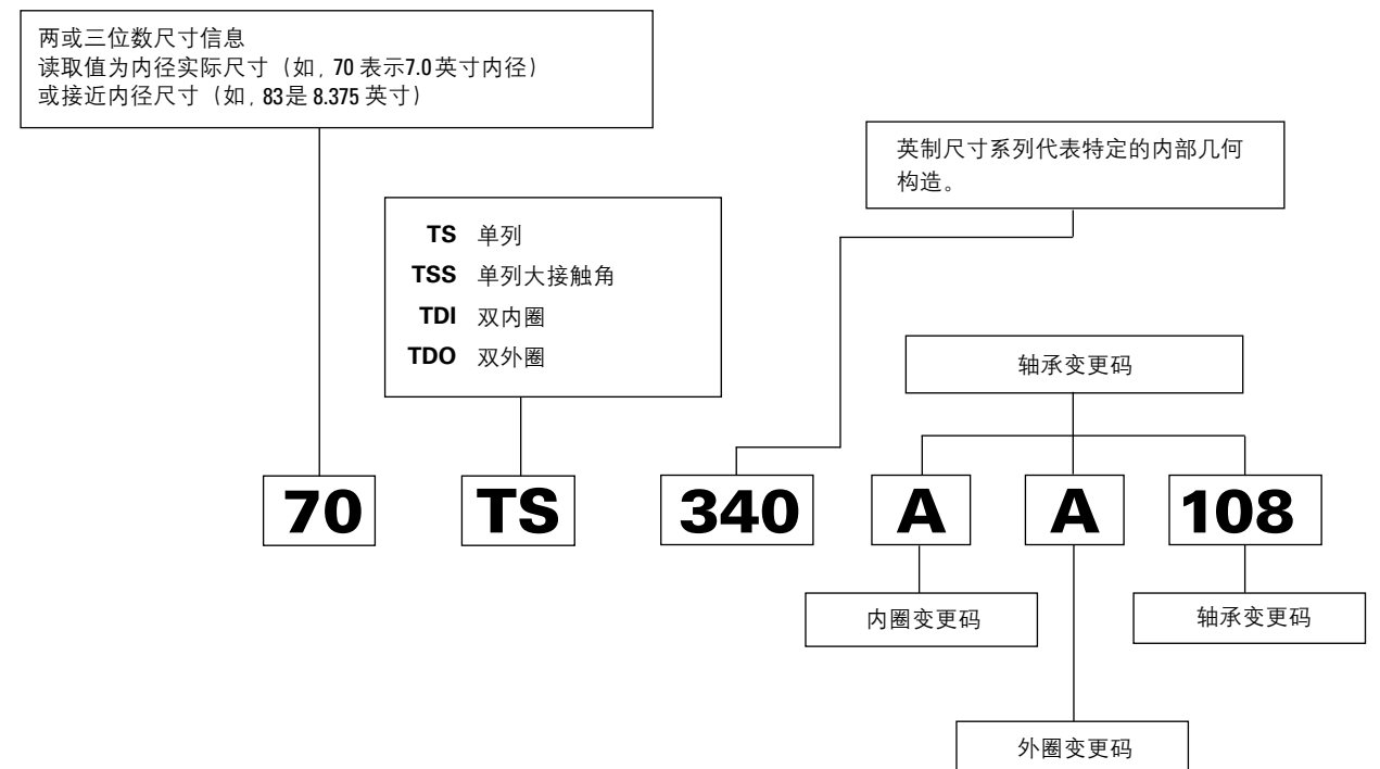
图 33. 圆锥滚子轴承历史命名法
