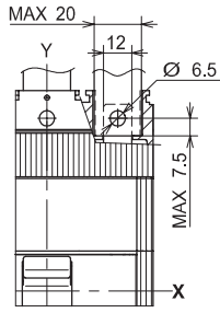
前接线端子 - F
