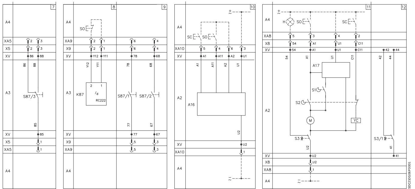
剩余电流脱扣器和遥控
