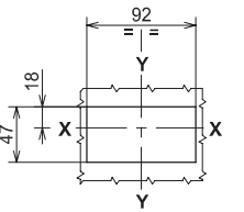
3 极 (不带法兰和断路器扩展)
