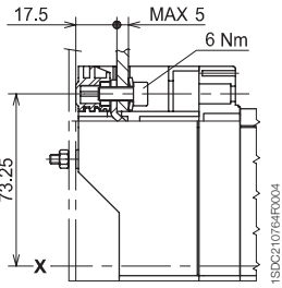
铜 / 铝电缆前接线端子 - FC CuAl 185mm 2
