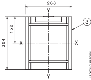
小室门法兰 (标配)
