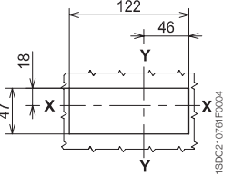
4 极 (不带法兰和断路器扩展)
