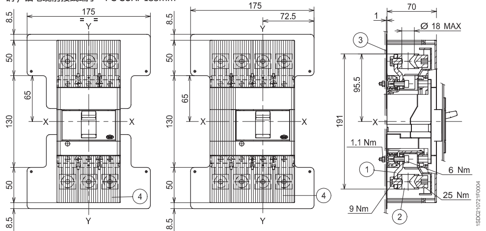
铜 / 铝电缆前接线端子 - FC CUI 185mm 2
