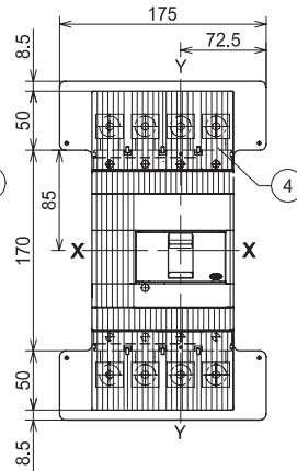
铜 / 铝电缆前接线端子 - FC CuAl 185mm 2
