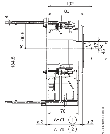
后水平接线端子 - HR
