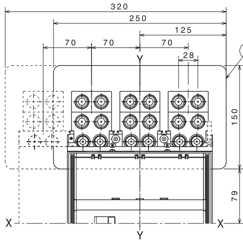
铜 / 铝电缆前接线端子 - FC CuAl 4 x 240 mm 2
