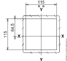
3-4 极 (带法兰)
