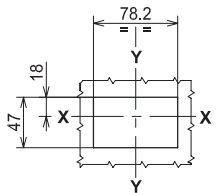
3-4 极 (不带法兰和断路器与小室门齐)
