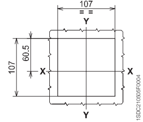
3-4 极 (不带法兰)
