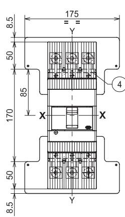
铜 / 铝电缆前接线端子 - FC CuAl 185mm 2
