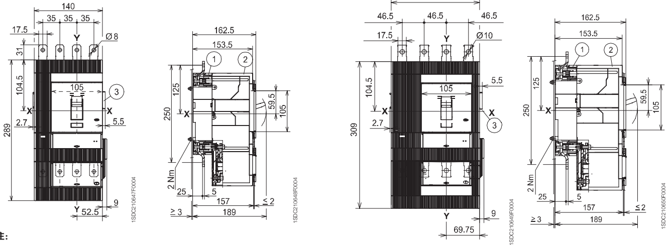
前接线端子 - F 安装在钢板上
