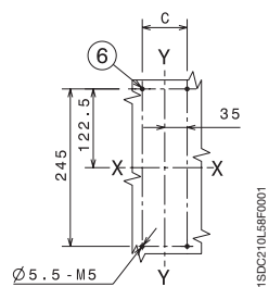
支撑钢板钻孔图
