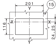
小室门钻孔图
