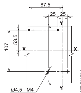
支撑钢板钻孔图
