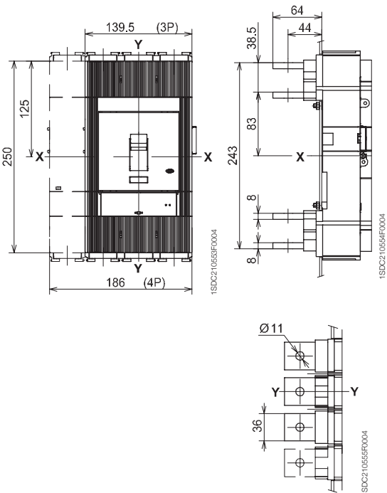
后水平接线端子 - HR 630 A
