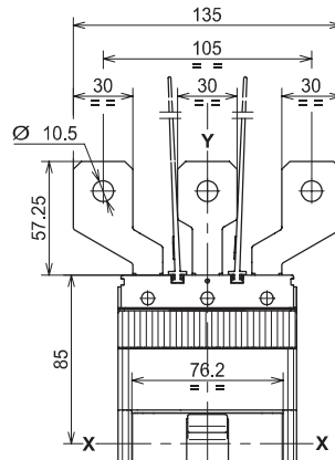
加长扩展型前接线端子 - ES
