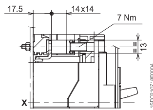
铜 / 铝电缆前接线端子 - FC CUI 185mm 2
