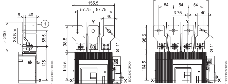
加长扩展型前接线端子 - ES 400 A
