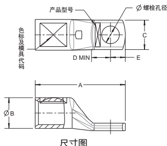
尺寸图
