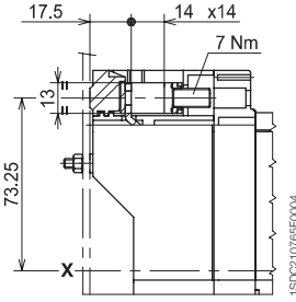
铜 / 铝电缆前接线端子 - FC CuAl 185mm 2
