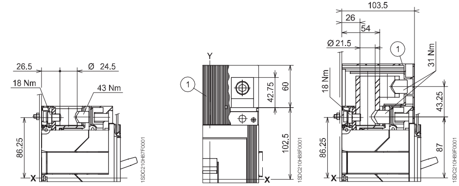
铜 / 铝电缆前接线端子 - FC CuAl 300mm 2
