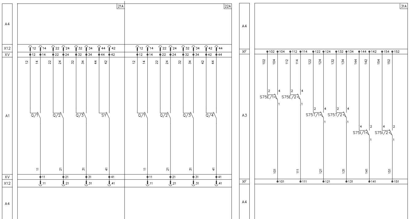
信号触头
