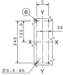
支撑钢板钻孔图
