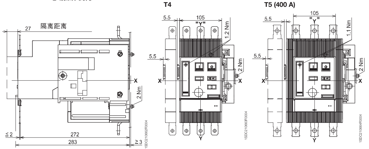
电动操作机构
