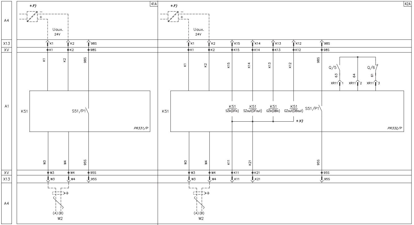
PR331/P和PR332/P电子脱扣器的辅助电路
