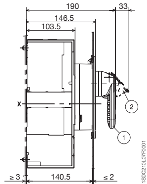
断路器旋转手柄操作机构
