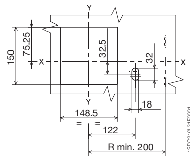
小室门钻孔图和安装法兰
