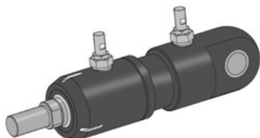
Befestigungsart 07 Mounting mode 07 Mode de fixation 07
