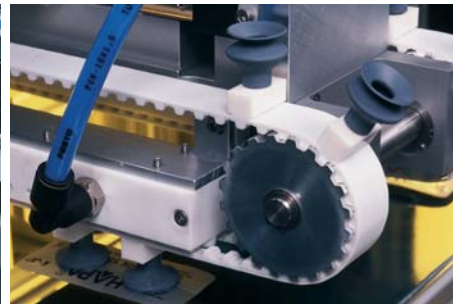
Fördervorrichtung für Blisterpackungen
