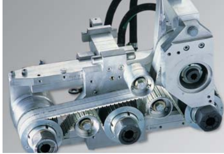
Dreifachbohrsystem
