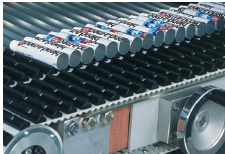
Tubenpackmaschine
