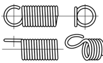
1/2 deutsche Öse
