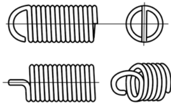
Haken eingerollt
