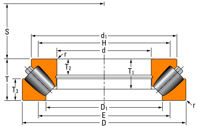
图 70. TSR-EM 型
