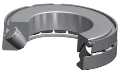
图 66. TSR-EJ 型
