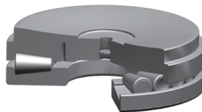
图 88. TTHDSV 型
