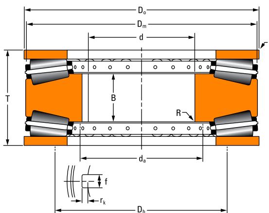
图 104. TTDK 1 型
