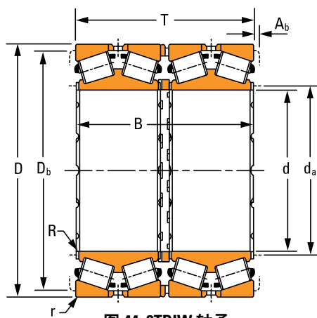
图 44. 2TDIW 轴承
