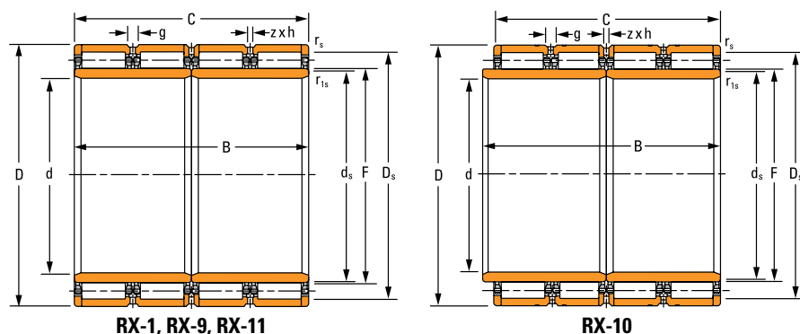
RX-1, RX-9, RX-11 表 49. 四列圆柱滚子轴承产品数据—接上页
