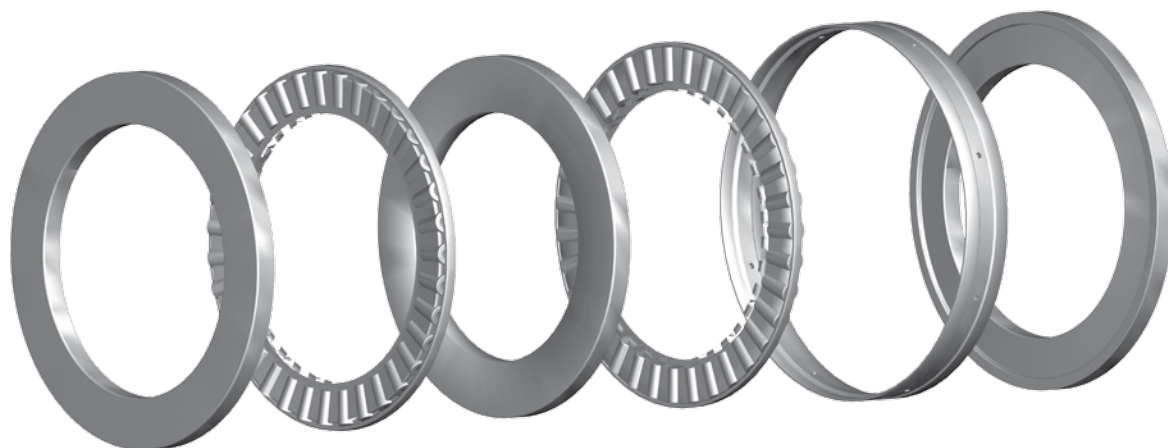
图 55. TTDFLK 轴承
