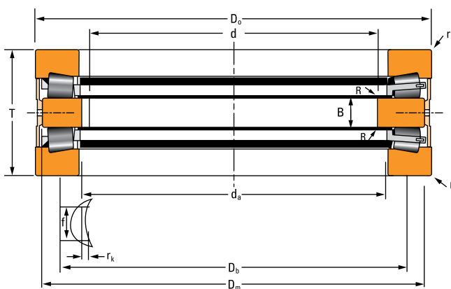
图 56. TTDFLK 轴承
