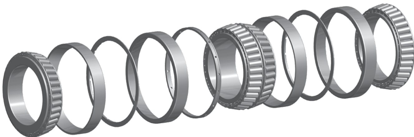
图 47. TQITS 轴承
