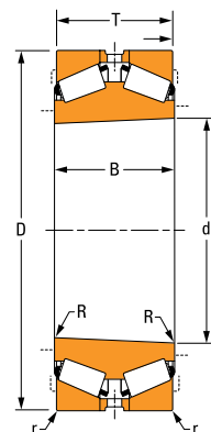
图 24. 圆锥滚子轴承 (TDIT 型)
