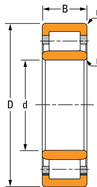
图 23. 圆柱滚子轴承
