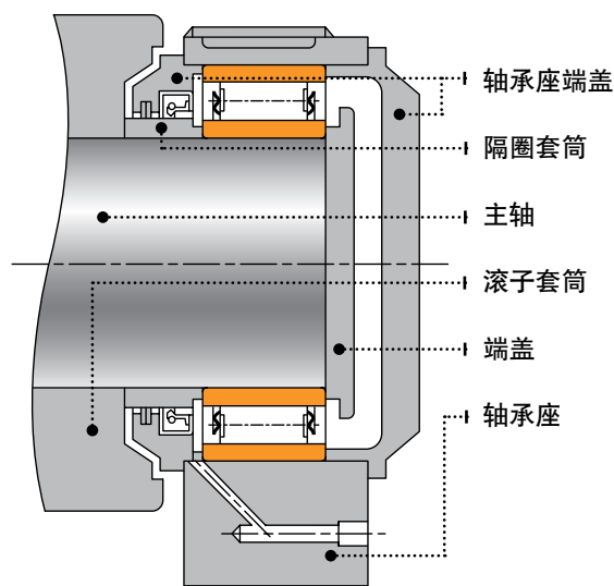
图 35. ADAPT 轴承
