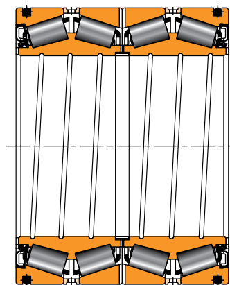
图 9. 密封辊颈轴承
