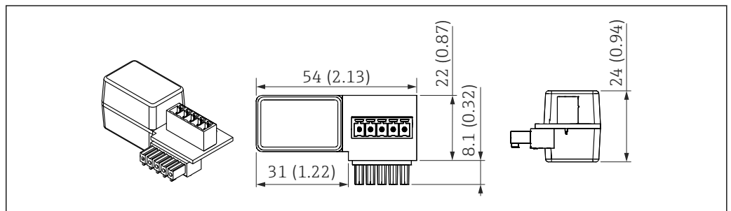
图 46 HART 通信电阻的外形尺寸; 单位: mm (in)
