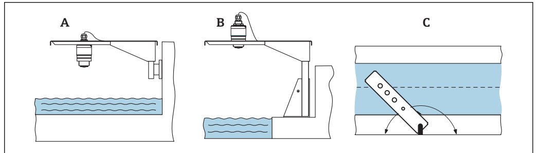
图 18 使用悬臂安装（可旋转）
