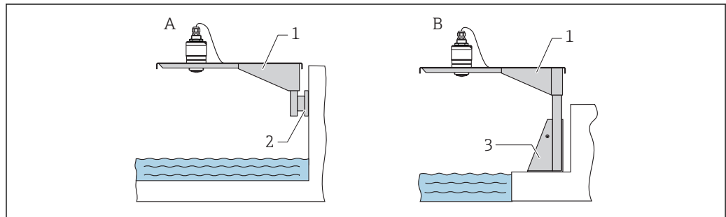
图 40 传感器过程连接（正面）的安装方式
