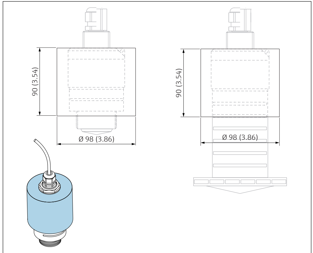
图 32 防护罩的外形尺寸；单位：mm (in)
