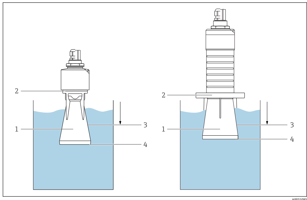
图 16 防浸没罩的功能示意图
