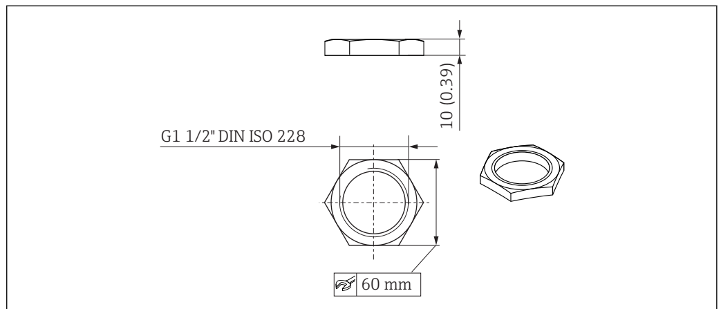
图 33 锁紧螺母的外形尺寸；单位：mm (in)
