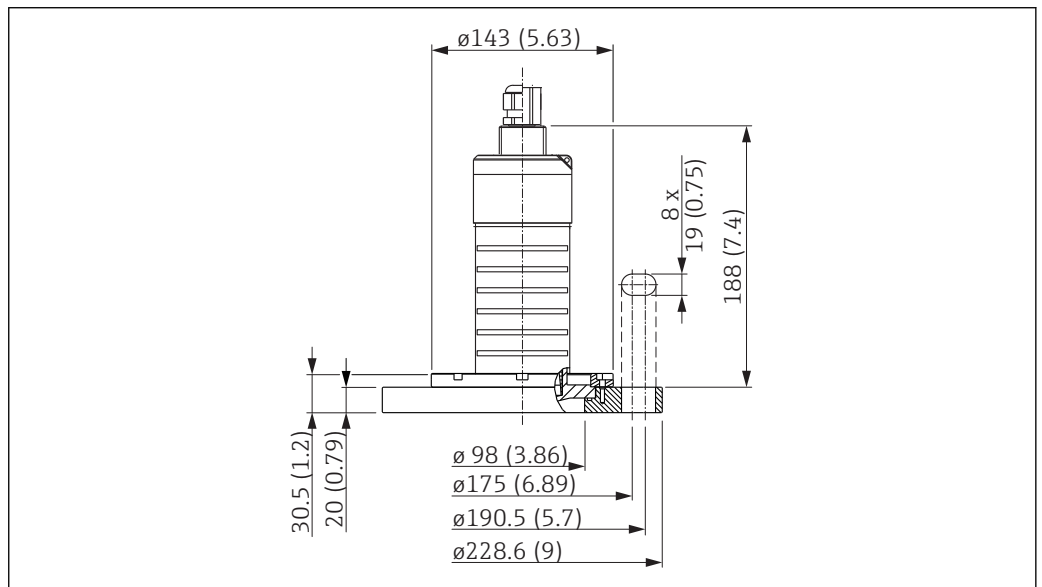
图 26 80 mm (3 in) 天线的外形尺寸，带 4"/DN100 松套法兰；单位：mm (in)
