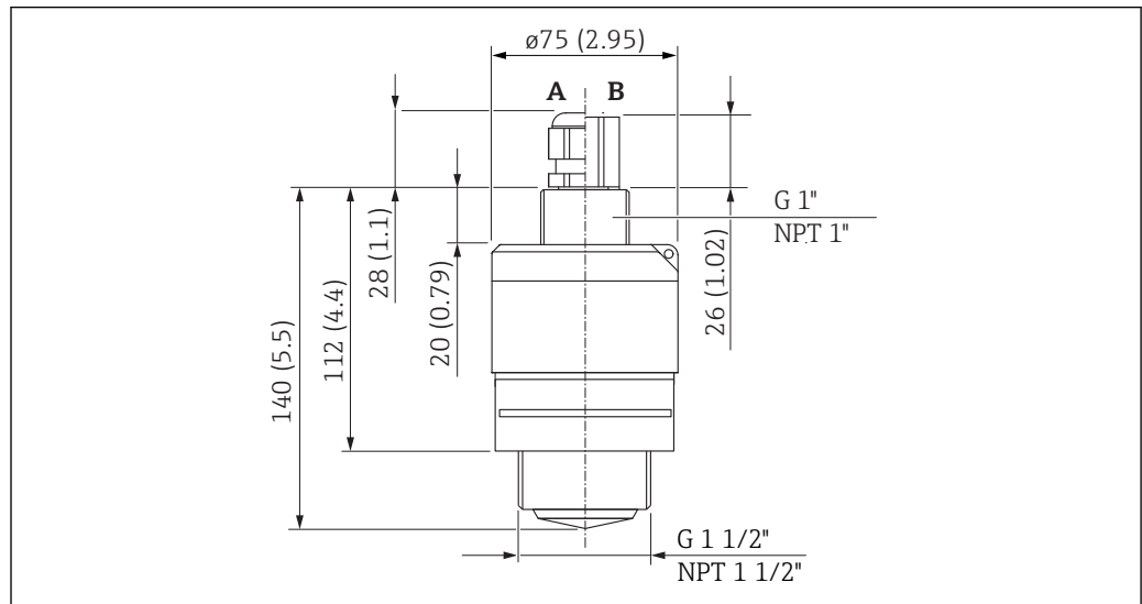
图 20 G 1-1/2" 或 MNPT 1-1/2" 螺纹过程连接的外形尺寸; 单位: mm (in)
