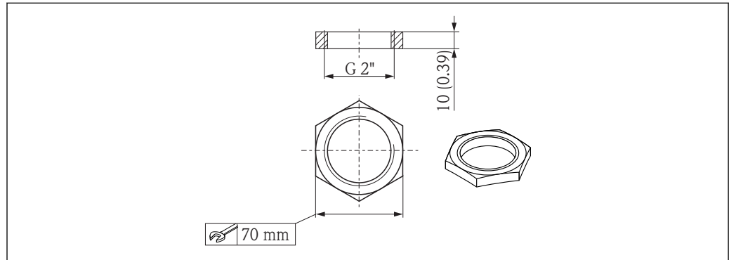
图 34 锁紧螺母的外形尺寸; 单位: mm (in)
