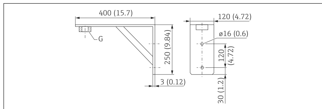
图 37 角型支架的外形尺寸; 单位: mm (in)
