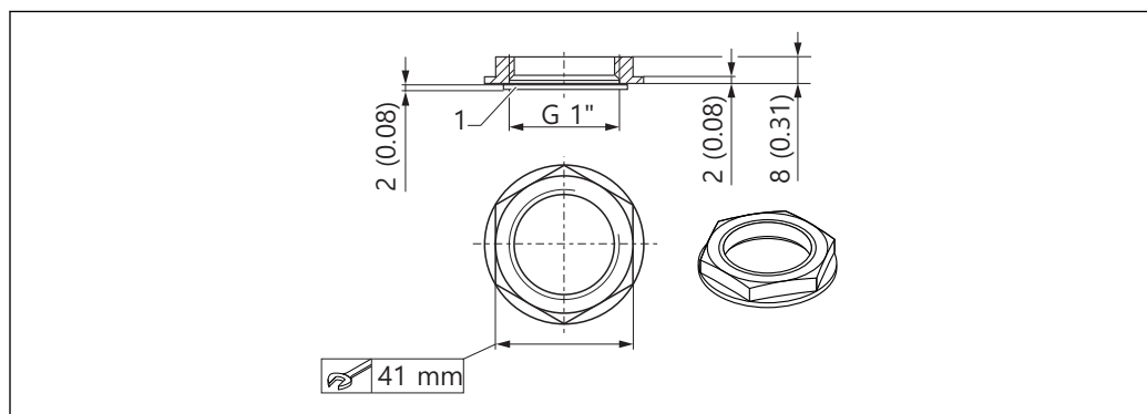
图 28 锁紧螺母的外形尺寸，适用于过程连接（背面）；单位：mm (in)
