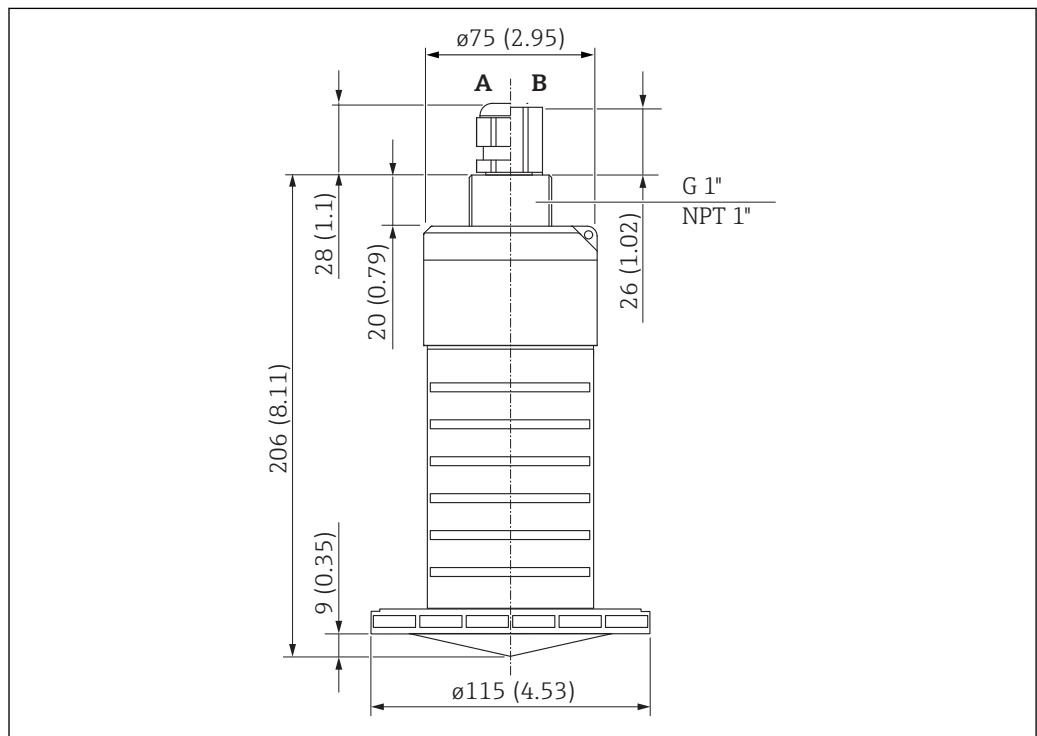
图 23 80 mm (3 in) 天线的外形尺寸; 单位: mm (in)
