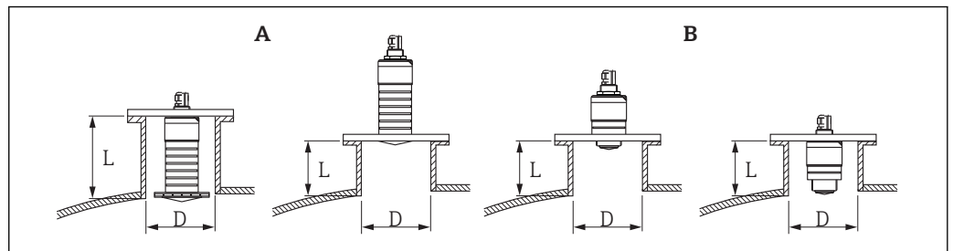
图 10 在安装短管中安装 FMR20
