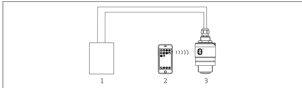
图 30 通过 Bluetooth®无线技术实现远程操作
