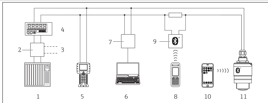
图 31 通过 HART 通信实现远程操作
