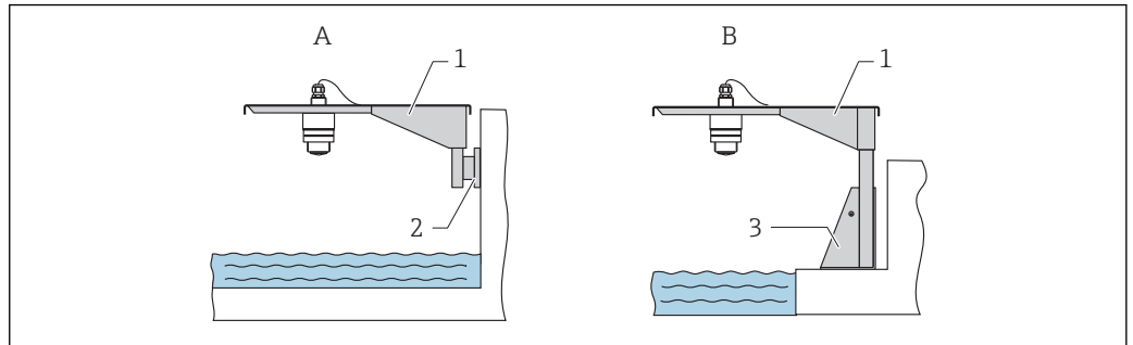
图 38 传感器过程连接（背面）的安装方式
