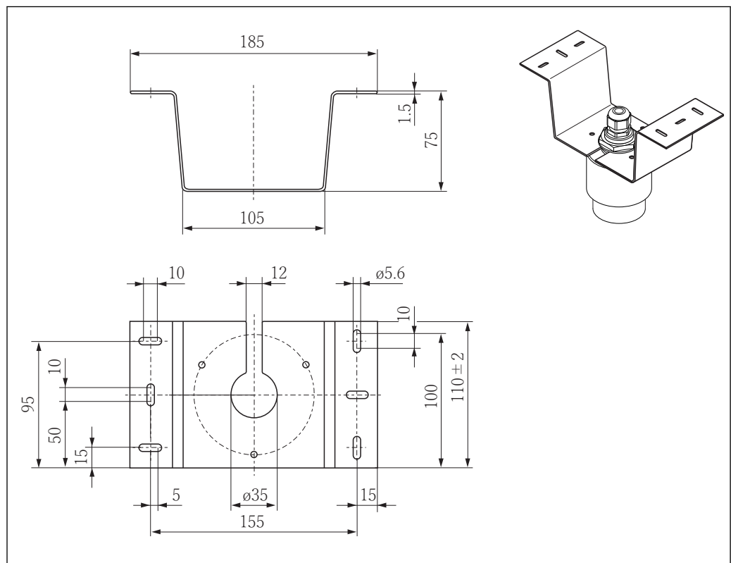
图 44 仓顶安装架的外形尺寸；单位：mm (in)
