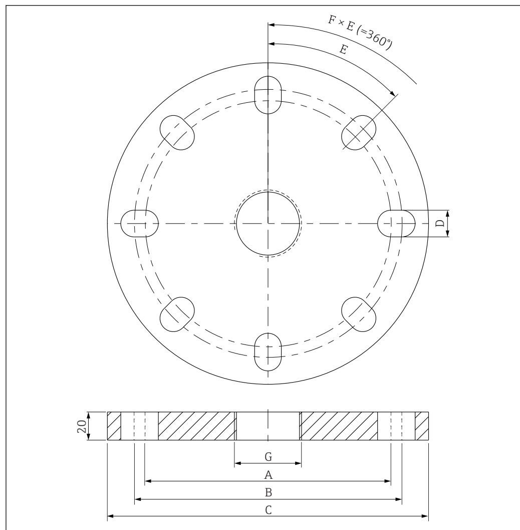
图 36 UNI 法兰的外形尺寸; 单位: mm
