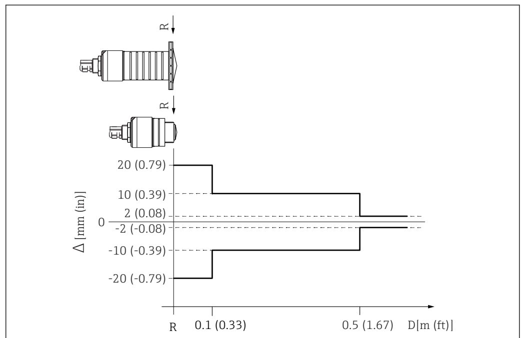
图 8 近距离测量时的最大测量误差; 图示为标准型仪表的数值
