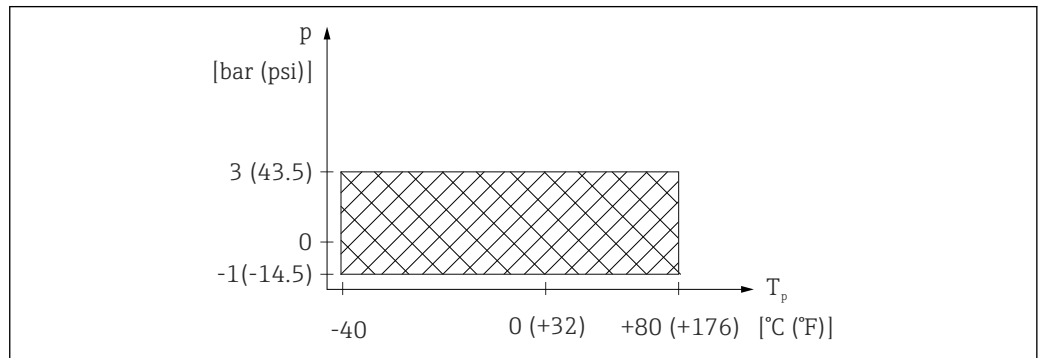
图 19 FMR20: 允许过程温度和过程压力范围
