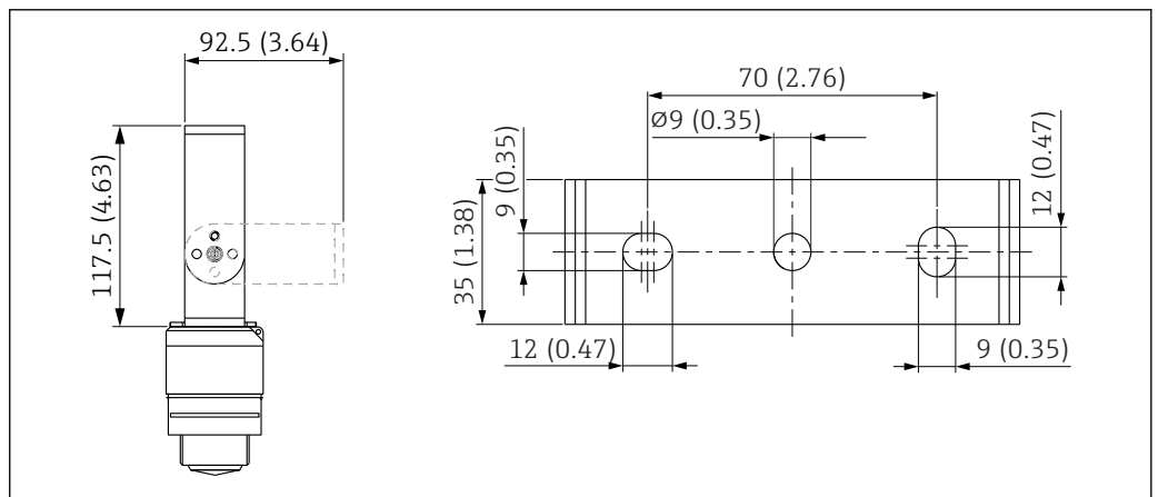
35 墙装支架的外形尺寸; 单位: mm (in)
