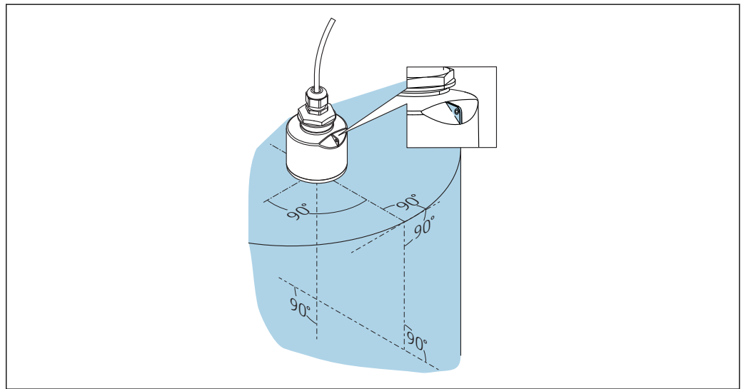
12 罐体中的传感器安装方向
