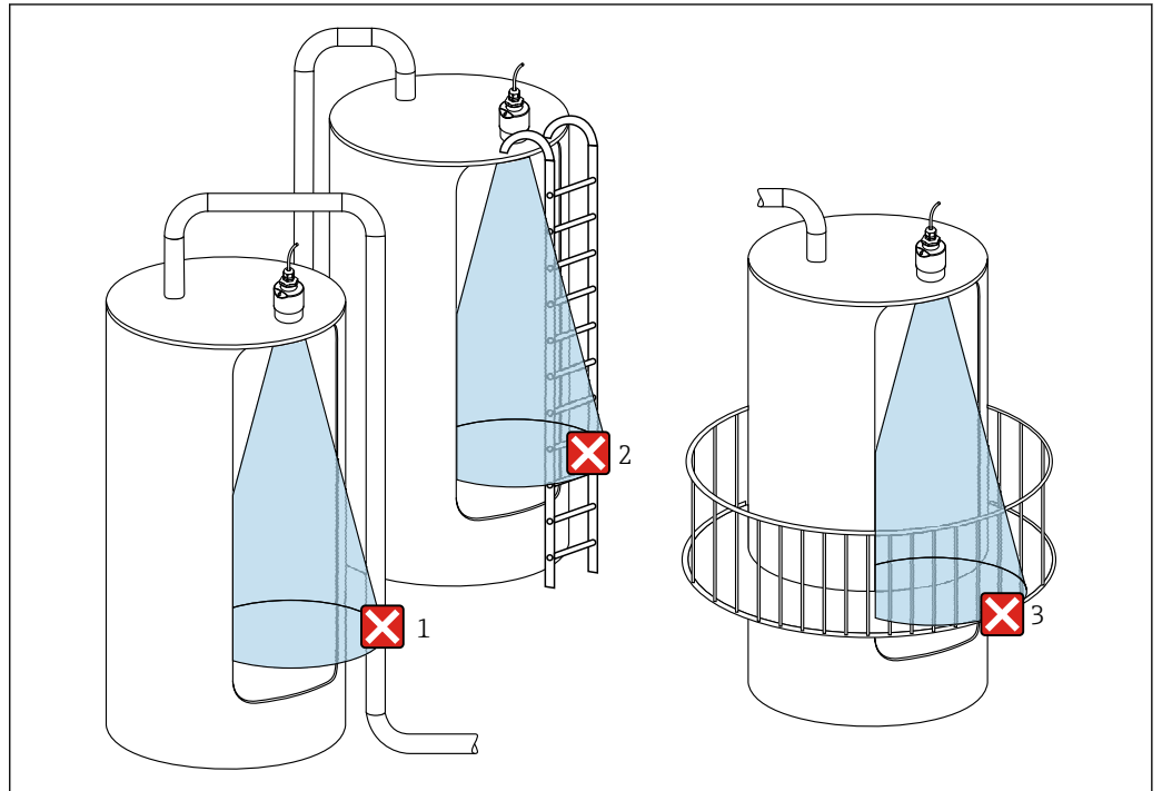
图 14 在塑料罐中测量
