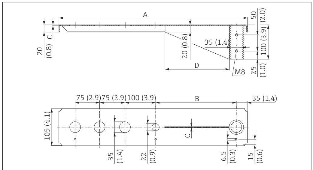
图 39 传感器过程连接（背面）安装的旋转悬臂的外形尺寸；单位：mm (in)
