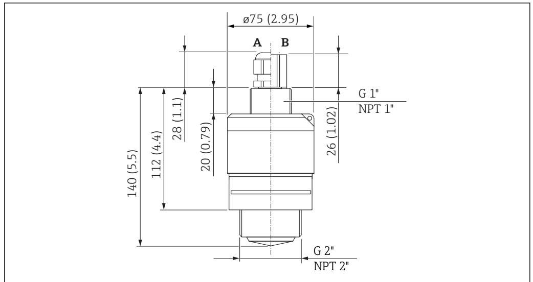
图 21 G 2" 或 MNPT 2" 螺纹过程连接的外形尺寸; 单位: mm (in)
