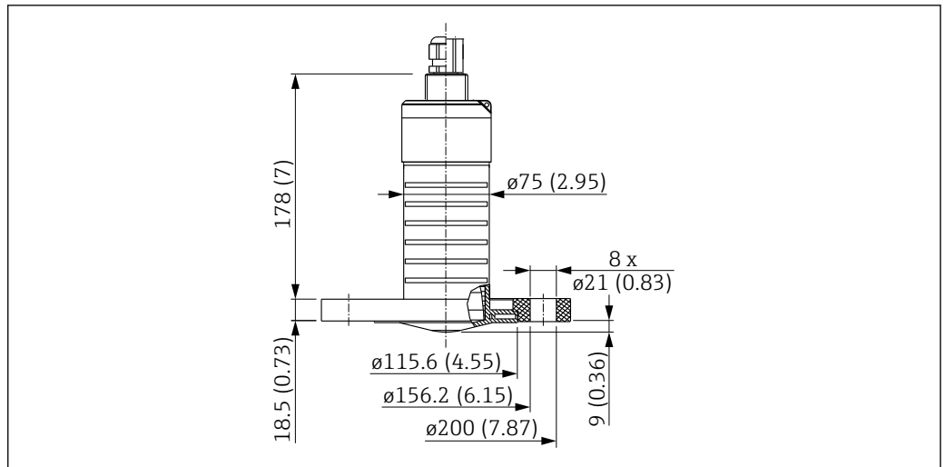
图 25 80 mm (3 in) 天线的外形尺寸，带 3"/DN80 松套法兰；单位：mm (in)
