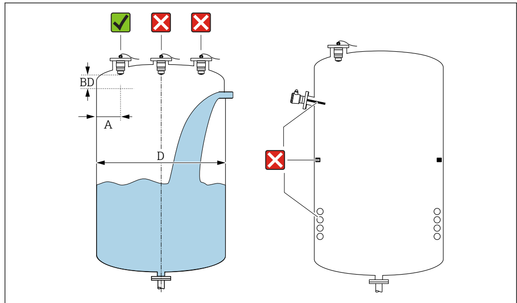
图 11 在罐体上的安装位置
