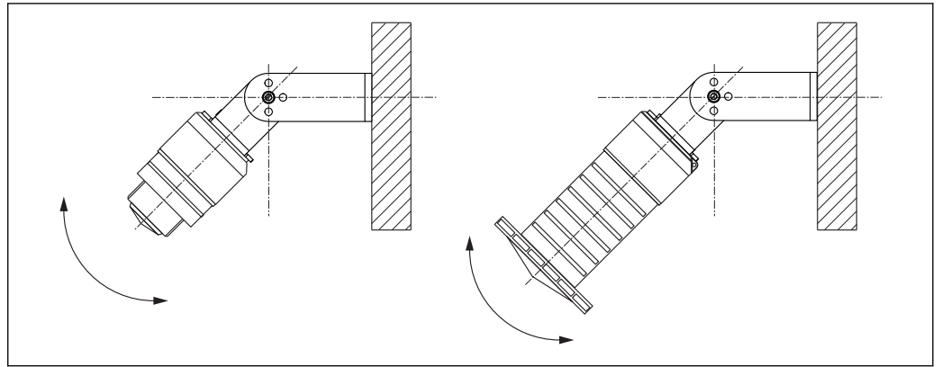
图 17 使用墙装支架安装（可调节）
