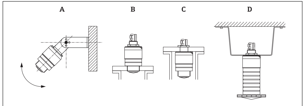
图 9 安装在墙壁上、罐顶上或安装短管中
