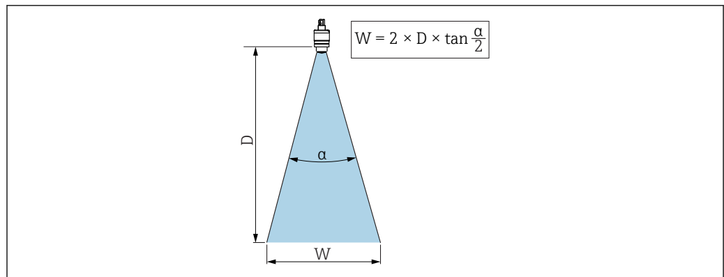
图 13 波束角 \alpha 、距离 D 和波束宽度 W 的相互关系
