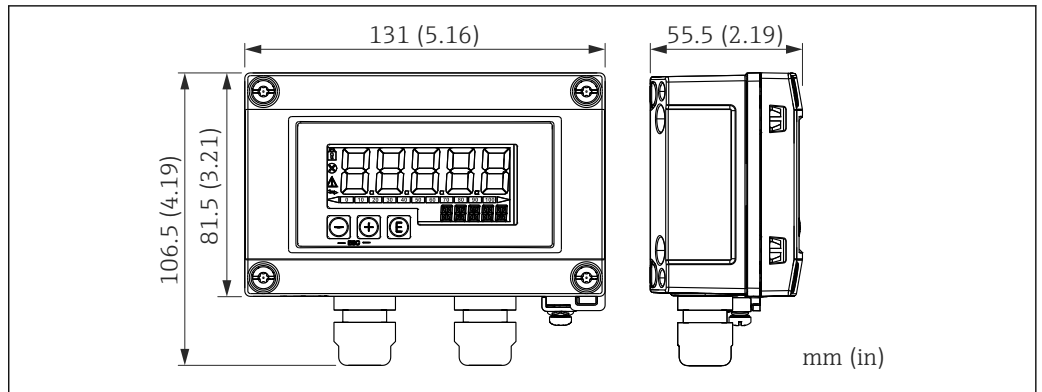
图 45 安装在现场型外壳中的 RIA15 的外形尺寸; 单位: mm (in)
