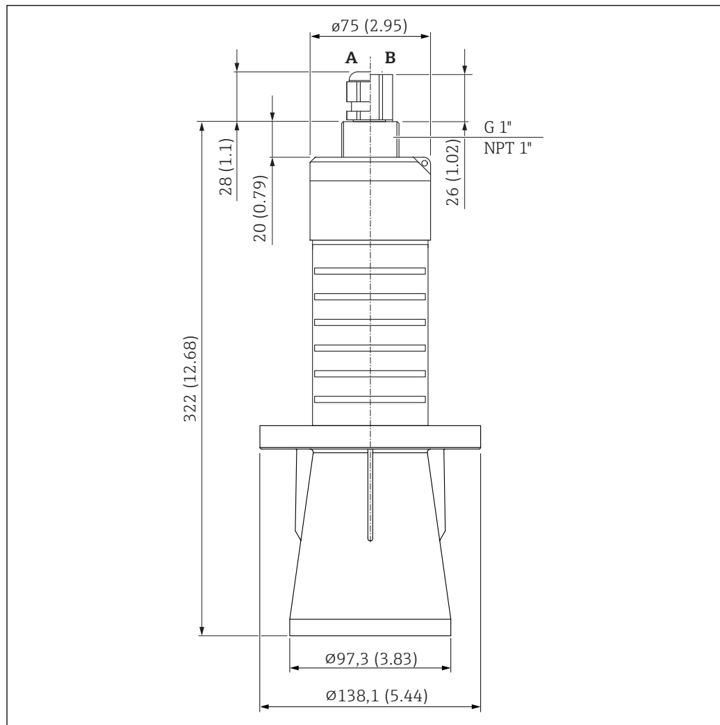
图 24 80 mm (3 in) 天线的外形尺寸，带防浸没罩；单位：mm (in)
