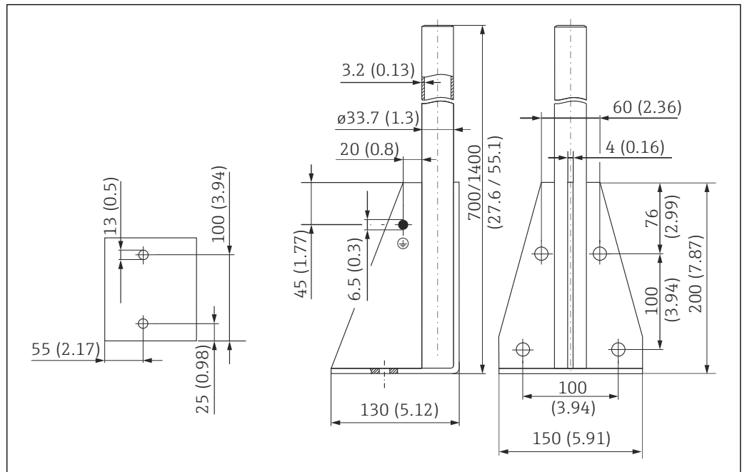
图 42 安装架的外形尺寸示意图; 单位: mm (in)
